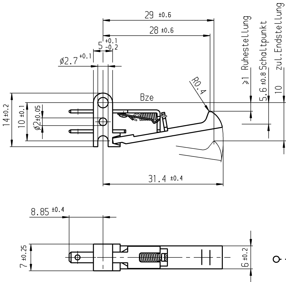
Flachstecker DIN 46 244-A 2,8-0,8 (EN 61058 / EN 61210)
